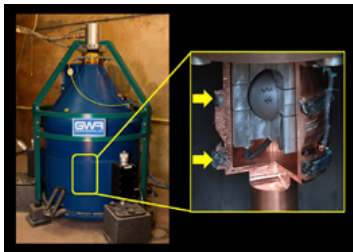
Figure 1 : à gauche le gravimètre à supraconductivité de Membach. L'encart montre la sphère, entourée de deux bobinages, indiqués par les deux flèches, où circulent les courants qui la font léviter (il s'agit ici d'un éclaté du capteur de l'ancien instrument d'Uccle, déclassé en 2000) (crédit : E. Coveliers (g), B. Frederick (d)).
